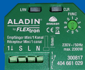
Récepteur ALADIN mini, 230 V, 1 canal, ENC No. d'art. 300817 E-No. 404 661 029
