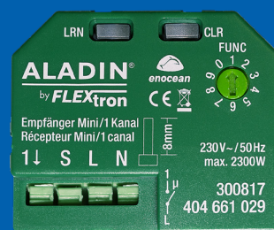
ALADIN Empfänger Mini, 230 V, 1 Kanal, UP Art.Nr. 300817 E-Nr.: 404 661 029
