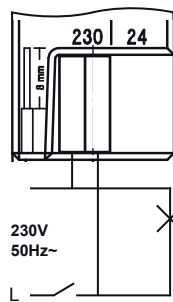
Beispiel Lampenschaltung
