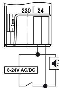
Beispiel Klingelschaltung
